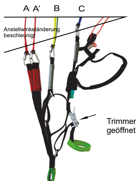
Stellung Trimmer offen
