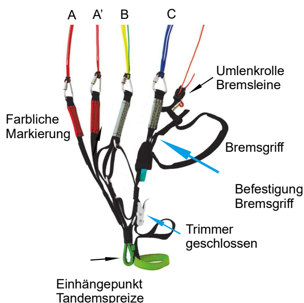
Stellung Trimmer geschlossen
