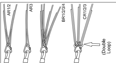
Werksauslieferung mit doppeltem Loop der BR4 und C-Stammleinen für die Trimmung bei Alterung
